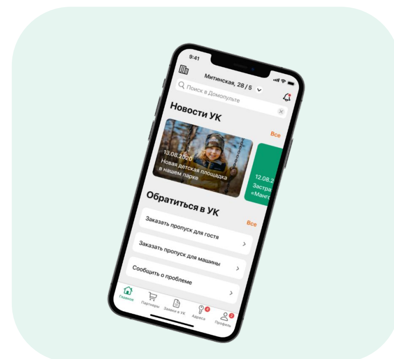
Приложение жителя
