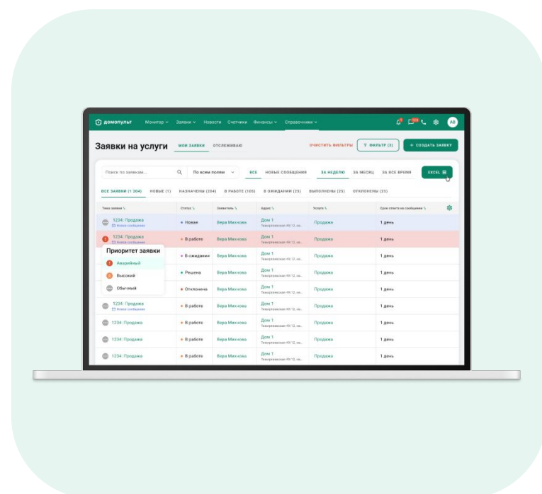
Кабинет Диспетчера
