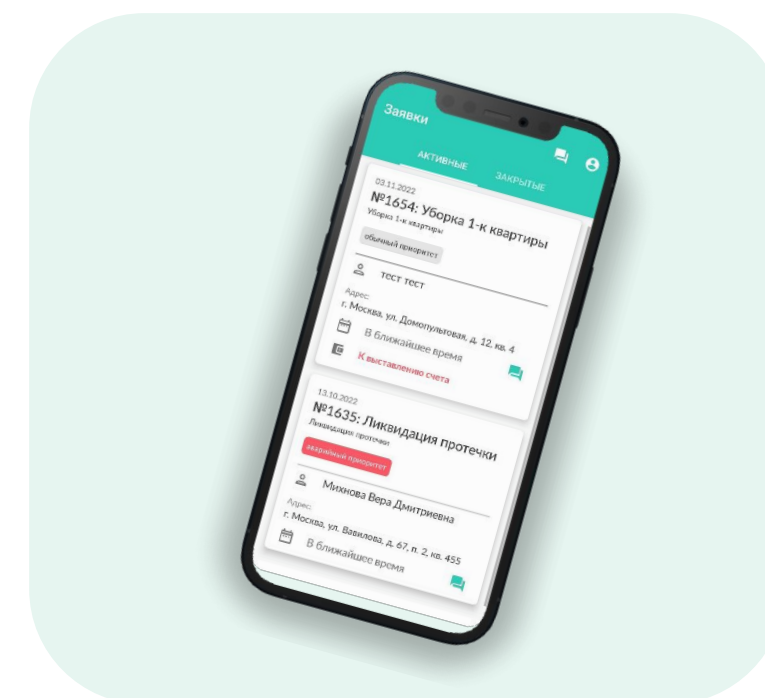
Приложение мастера
